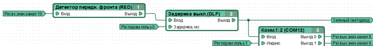
Рисунок 2.20 – Пример диаграммы для использования параметров пользовательской конфигурации.
