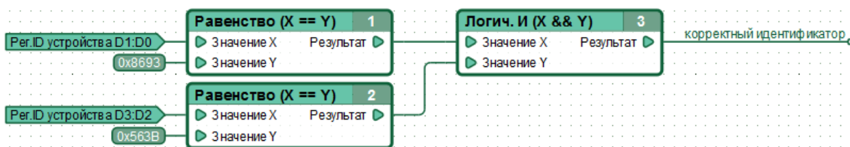
Рисунок 2.17 – Пример функциональной диаграммы, иллюстрирующей работу с идентификатором устройства.
