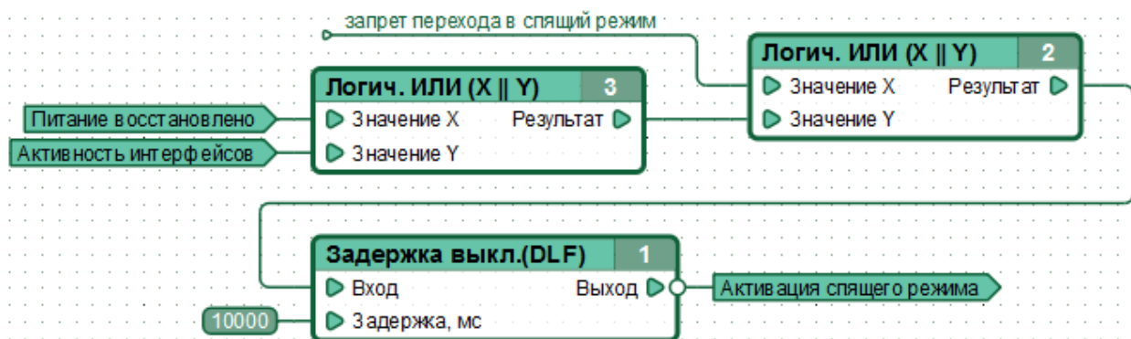
Рисунок 2.14 – Фрагмент функциональной диаграммы, реализующий типовое управление режимом пониженного энергопотребления: переход в режим пониженного энергопотребления в отсутствие в течение 10 секунд условий препятствующих этому и автоматический возврат в нормальный режим при активности периферии контроллера или по установке запрета «засыпания» из диаграммы.
