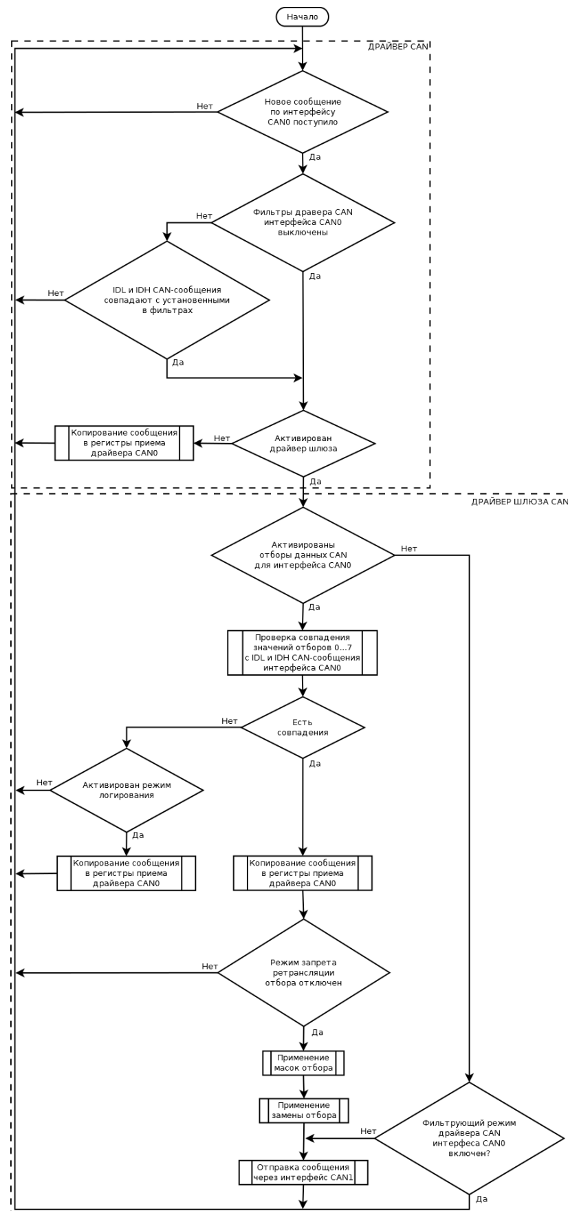
Рисунок 2.9 – Блок-схема работы контроллера в режиме CAN-шлюза.
