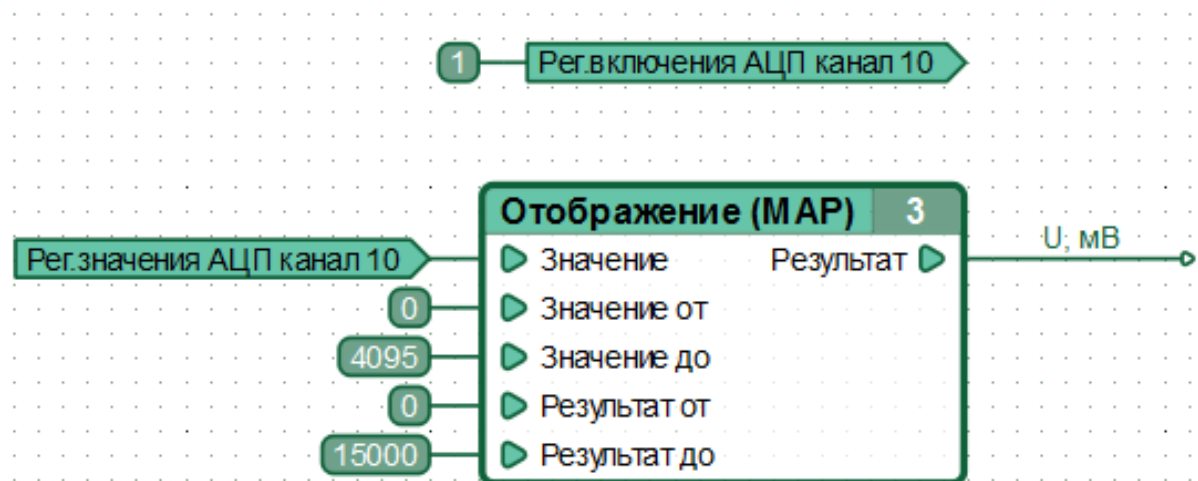
Рисунок 2.6 – Пример функциональной диаграммы активации АЦП канала №10 и получения результатов аналого-цифрового преобразования.
