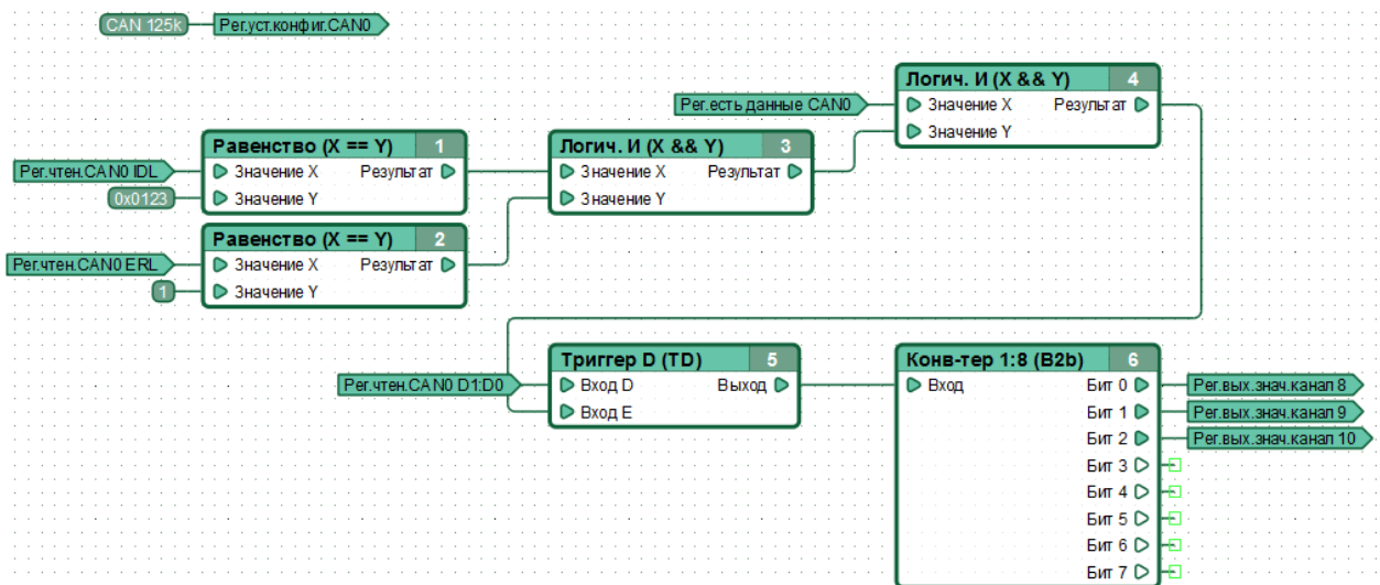
Рисунок 2.8 – Пример №2 функциональной диаграммы отправки данных в шину CAN через интерфейс CAN0.
