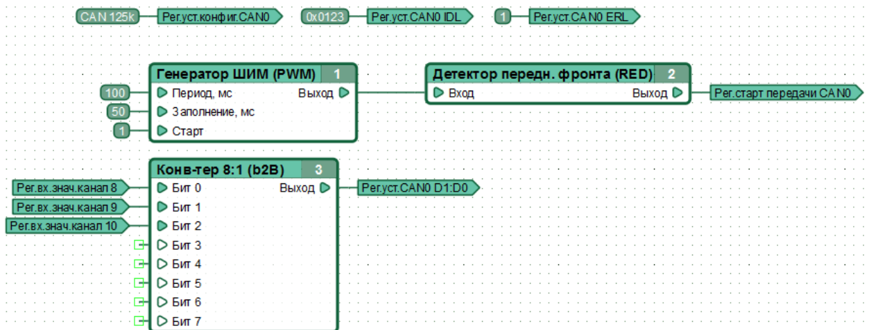
Рисунок 2.7 – Пример №1 функциональной диаграммы отправки данных в шину CAN через интерфейс CAN0.
