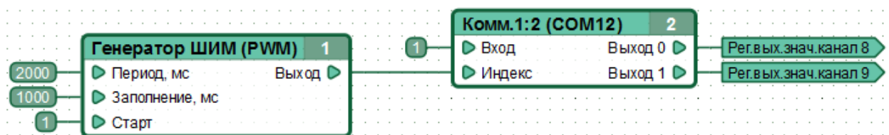
Рисунок 2.11 – Пример функциональной диаграммы выполняющей ежесекундное поочередное переключение электрических потенциалов с «+12В»(1мА) на «GND»(100мА) на контактах контроллера, соответствующих каналам №8 и №9.
