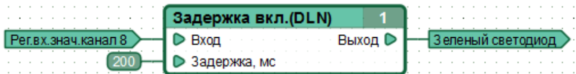
Рисунок 2.12 – Пример функциональной диаграммы, включающей встроенный зеленый светодиод контроллера при поступлении и удержании в течение не менее 200мс на соответствующем канале №8 контакте контроллера, потенциала GND.
