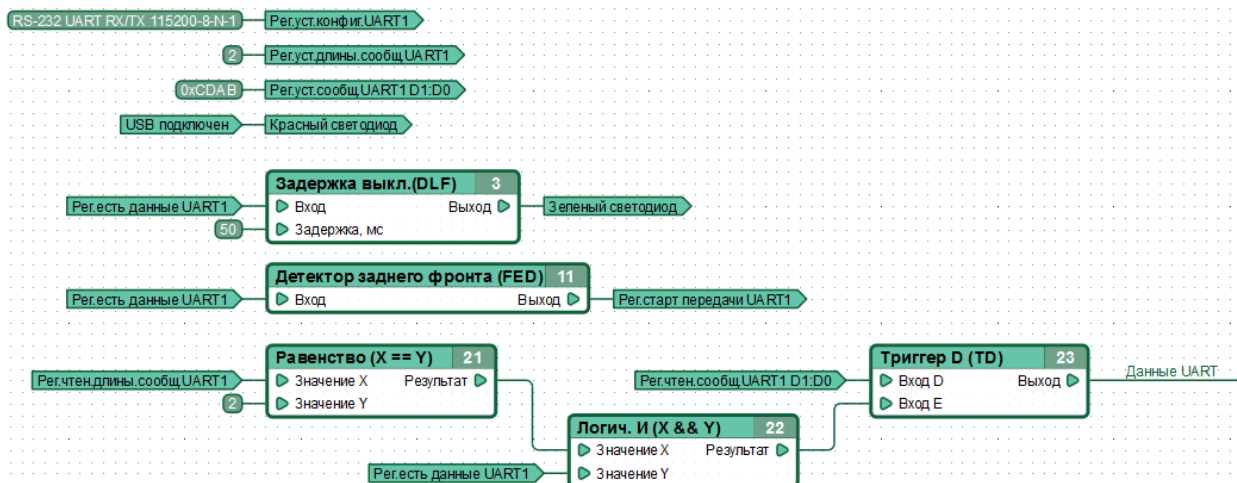
Рисунок 2.19 – Диаграмма подключения
