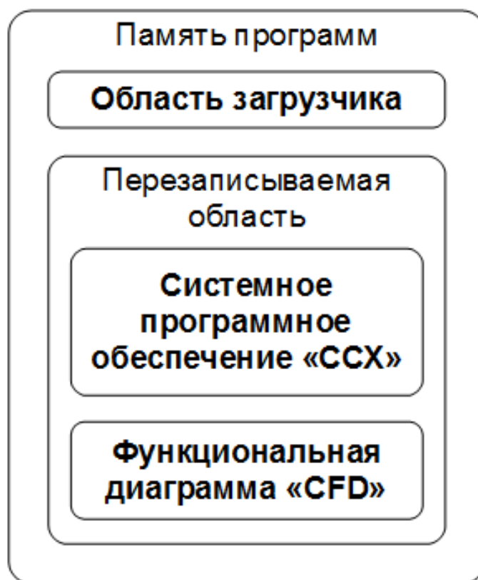
Рисунок 2.5 – Структура программного обеспечения контроллера CANNY 5.2 duo
