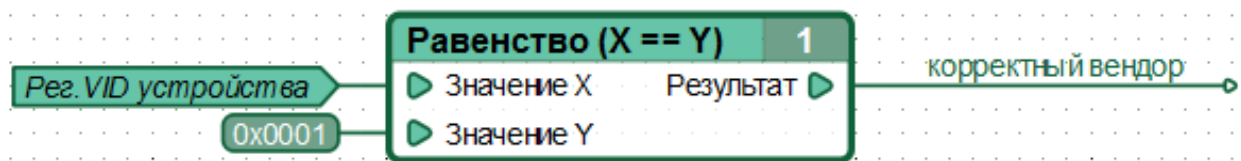
Рисунок 2.18 – Пример функциональной диаграммы, иллюстрирующей работу с идентификатором вендора устройства.
