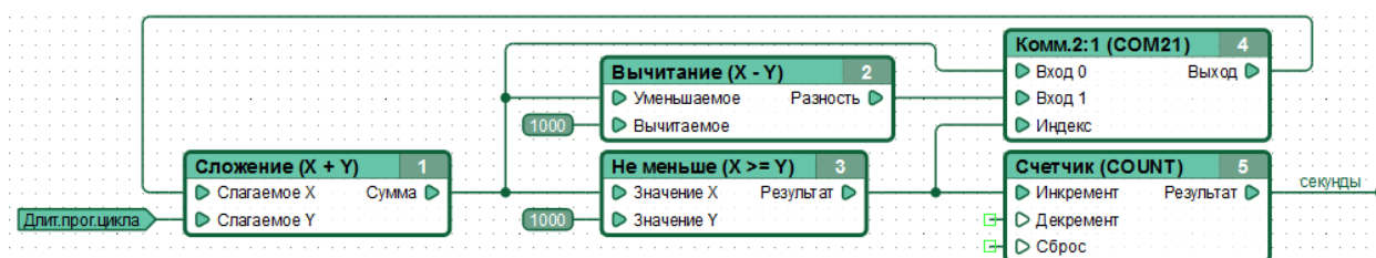
Рисунок 2.16 – Фрагмент функциональной диаграммы, реализующий высокоточный счетчик секунд, пригодный для использования в часах реального времени.
