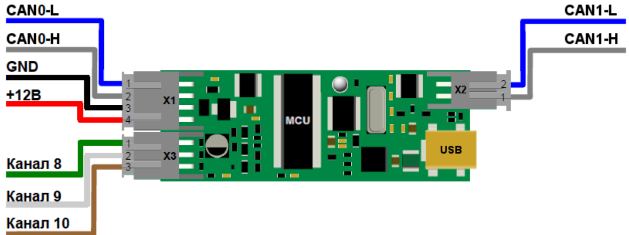
Рисунок 2.2 – Схема контроллера CANNY 5.2 duo
